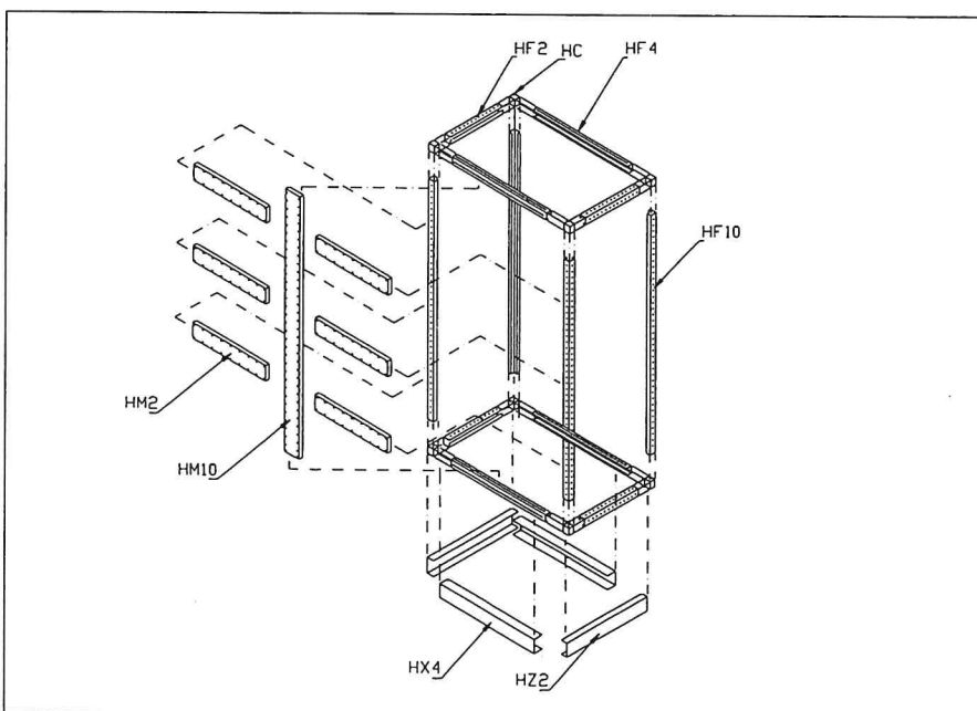
Assembling of [2 modules x 4 modules x 10 modules] cubicle. (2 模数 x 4 模数 x 10 模数) 的组装图。
