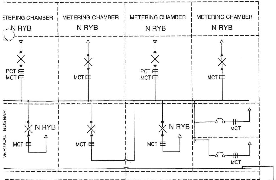
BUSBAR ARRANGEMENT 母线排位
