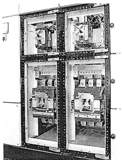
250A and 800A MCCB installation in the panel. 250A 及 800A MCCB 开关小室。
