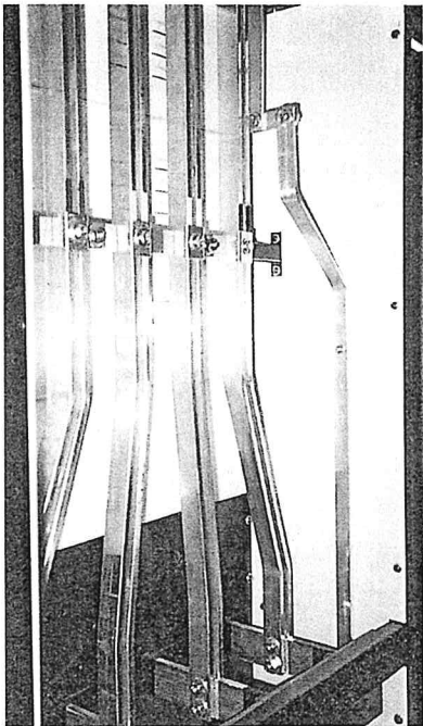
Busbar connect to Transformer. 由开关柜连接至变压器的母线。
