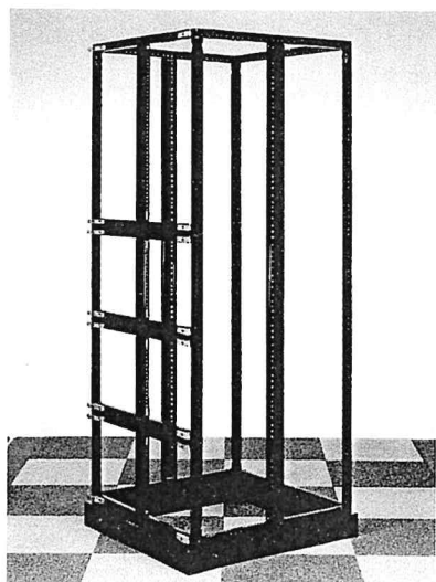
Base frame arrangement [4 modules x 4 modules x 10 modules]. 基本框架 (4 模数 x 4 模数 x 10 模数)。
