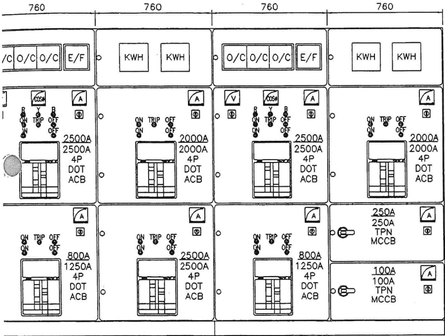
FRONT VIEW 正视图
