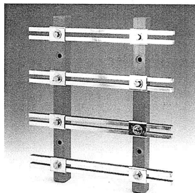
800A ~ 1250A Busbar Support. 800A ~ 1250A 母线。
