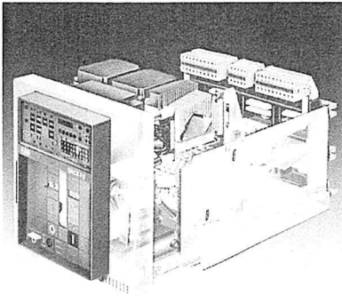
'ABB SACE' - Megamax ACB ABB SACE - Megamax F 系列空气断路器
