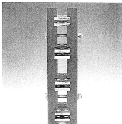
1600A and above Busbar support. 1600A 以上的母线。
